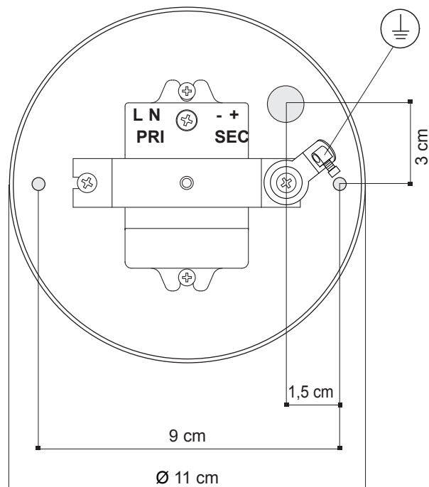
Schema per il fissaggio a plafone Outline for ceiling fitting
