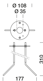
8950120 Tie-rod Ø 108 x D. 290
