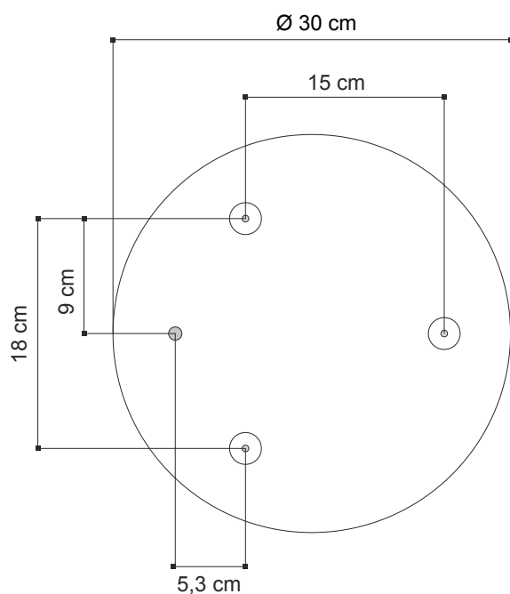
Schema di fissaggio a parete/plafone Outline for wall/ceiling fitting
