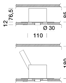
8945115 Recessed box E2 - drywall
