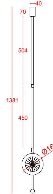
ÖN GÖRÜNÜŞ
