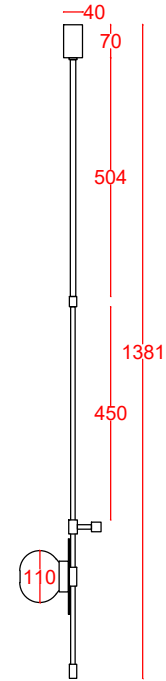
YAN GÖRÜNÜŞ
