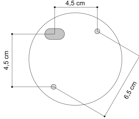
Schema per il fissaggio a plafone Outline for ceiling fitting
